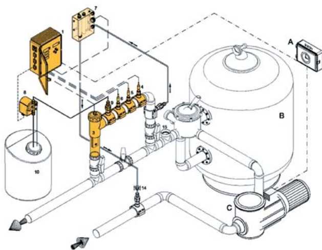
Esquema de instalação do sistema
